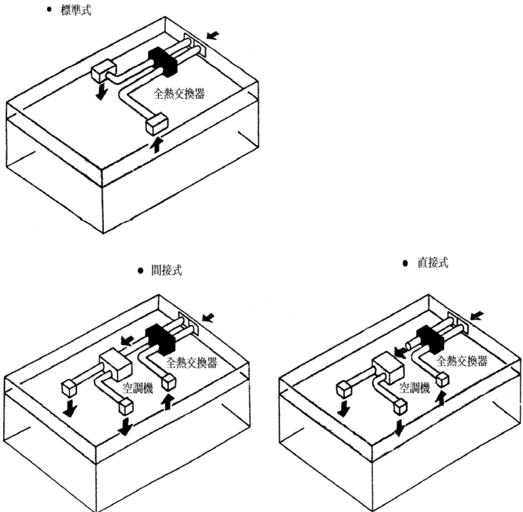
圖 4-5-11 全熱交換器安裝示意圖【13】
